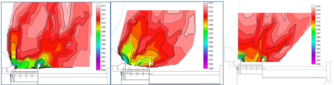
Figura 9.- Superficie digital del modelo cuando se espera la crecida con las compuertas cerradas sin aporte de sedimentos, con aporte de sedimentos manual y con aporte de sedimentos continuo respectivamente.
