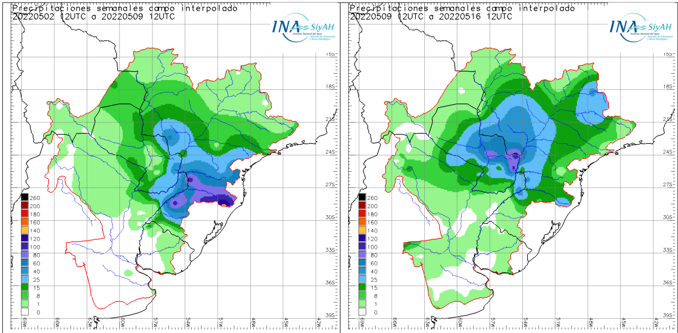
Lluvias semanales acumuladas al 09/may/2022
