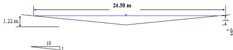
Figura 12.- Sección triangular mínima necesaria. Cauce Grande. TR=25 años
