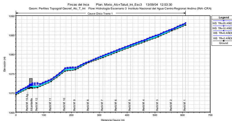
Figura 9.- Perfil Longitudinal Cauce Chico- TR=2,5,10 y 25 años
