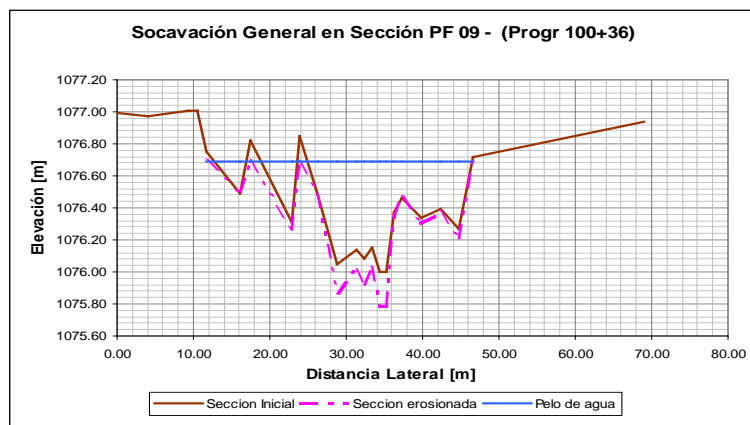
Figura 11.- Perfil Transversal Sección inicial y erosionada (PF09)
