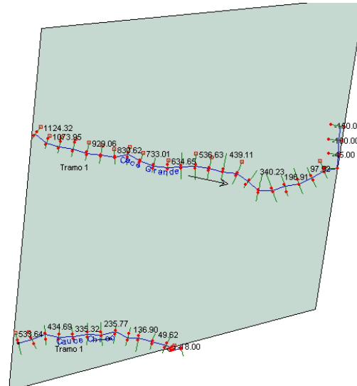
Figura 8.- Planimetría con ubicación de secciones transversales
