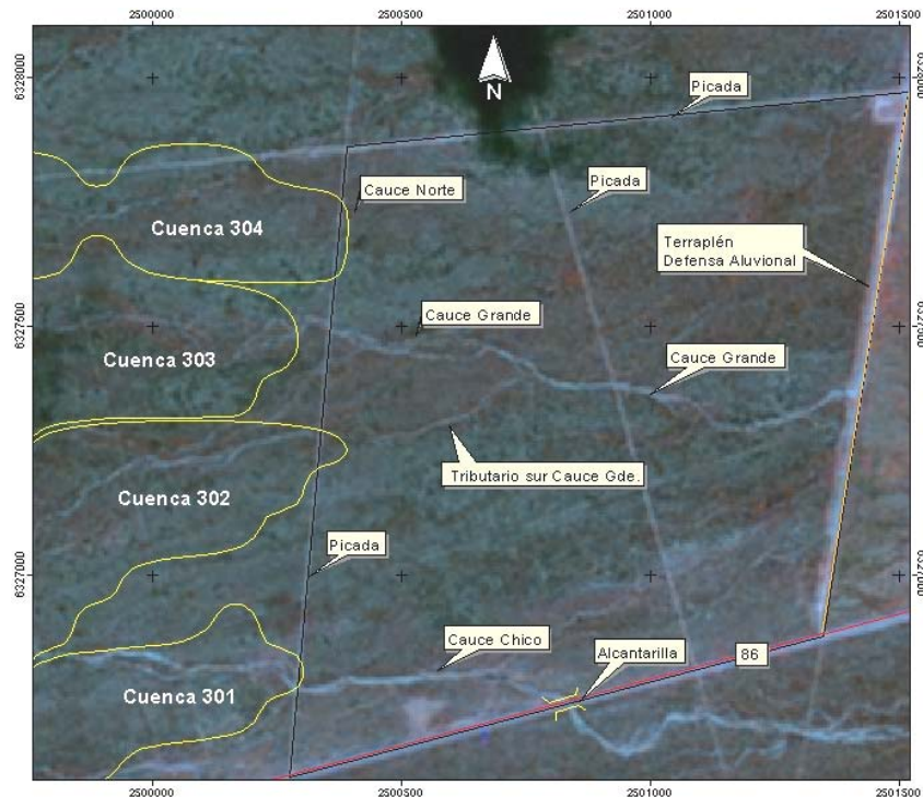
Figura 4.- Imagen satelital Ikonos
