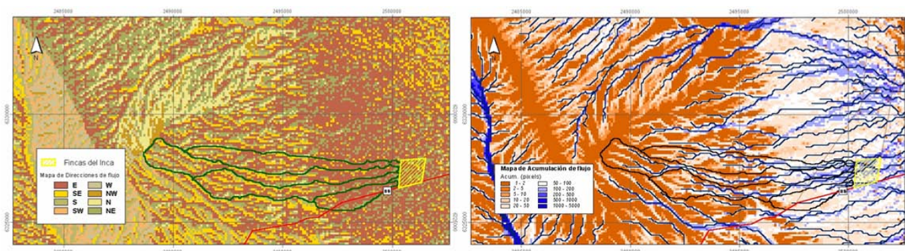
Figura 3.- Mapas de dirección y acumulación de flujo
