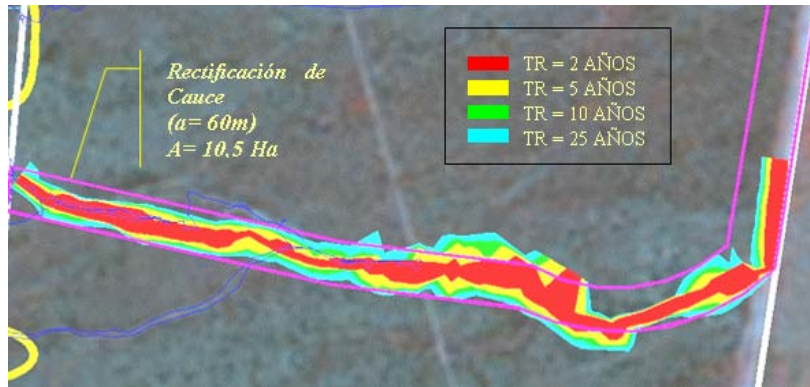
Figura 10.- Planicies de inundación para Cauce Grande
