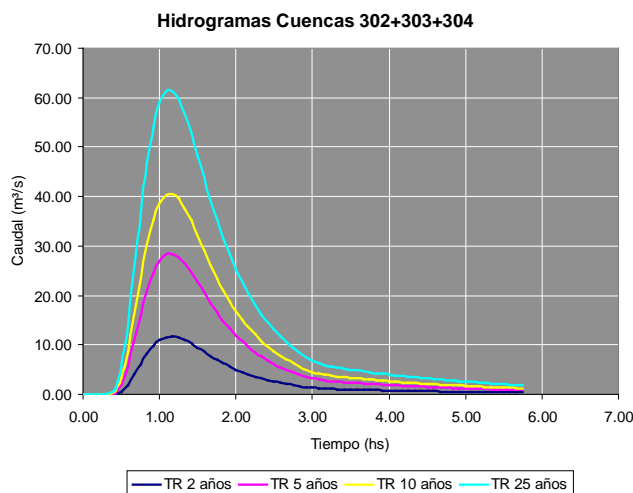
Figura 7.- Hidrogramas Nudo001. Escenario II
