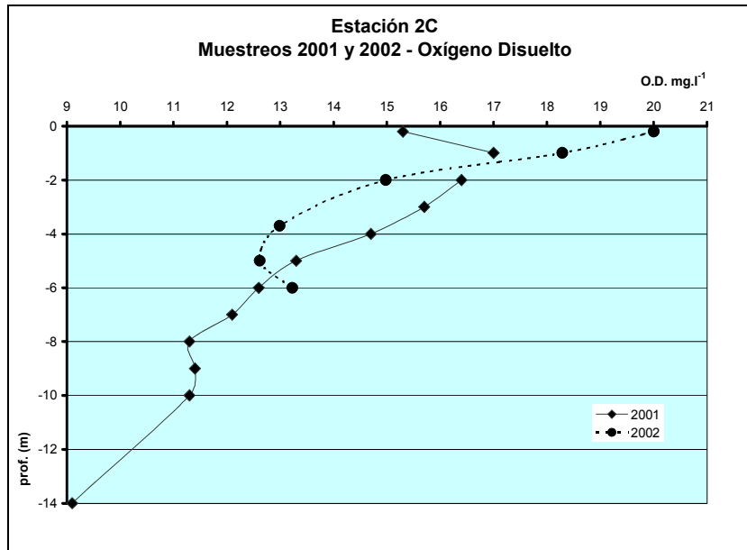
Figura 4. Oxígeno Disuelto. Estación 2C
