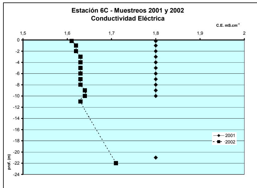
Figura 12. Conductividad Eléctrica. Estación 6C
