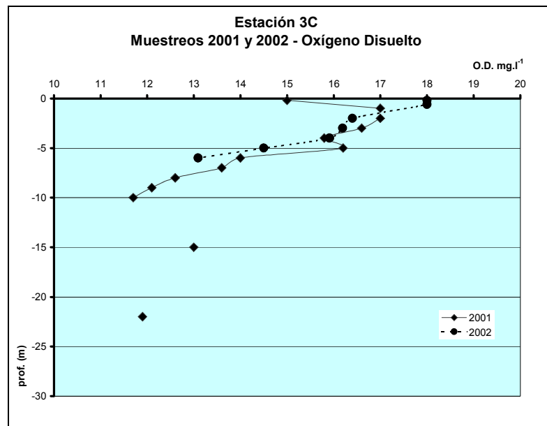
Figura 5. Oxígeno Disuelto. Estación 3C
