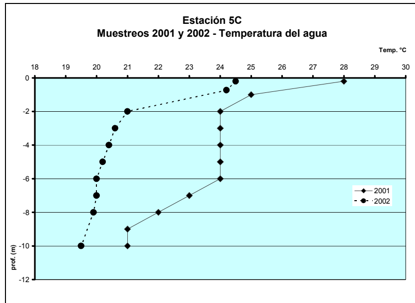
Figura 10. Temperatura del agua. Estación 5C
