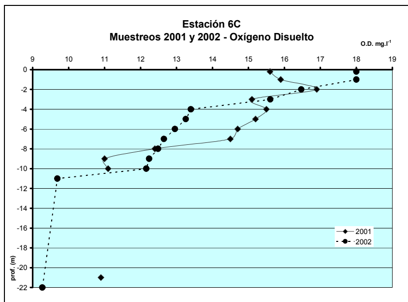
Figura 7. Oxígeno Disuelto. Estación 6C
