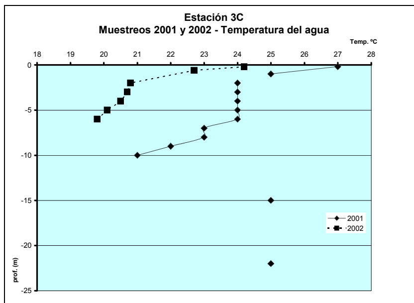
Figura 9. Temperatura del agua. Estación 3C
