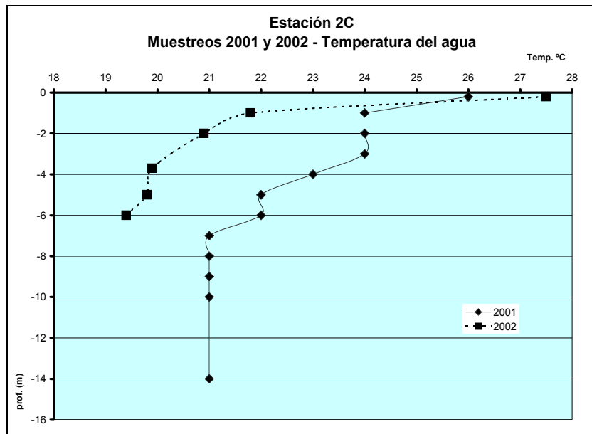
Figura 8. Temperatura del agua. Estación 2C
