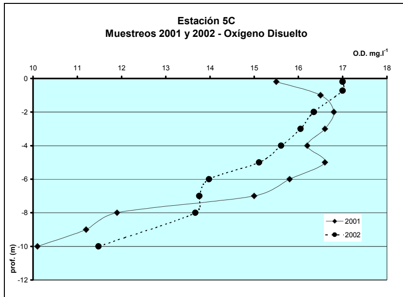
Figura 6. Oxígeno Disuelto. Estación 5C
