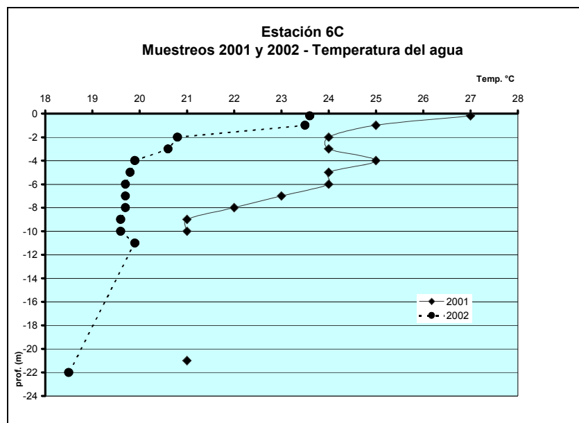
Figura 11. Temperatura del agua. Estación 6C
