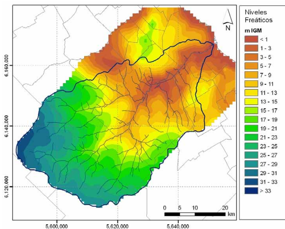
b) Con extracciones de grandes industrias
