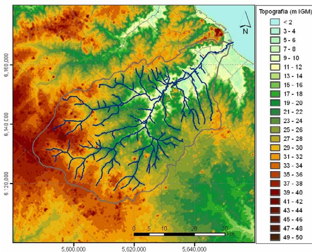
Figura 2.3.1. MDE para la Primera Etapa.
