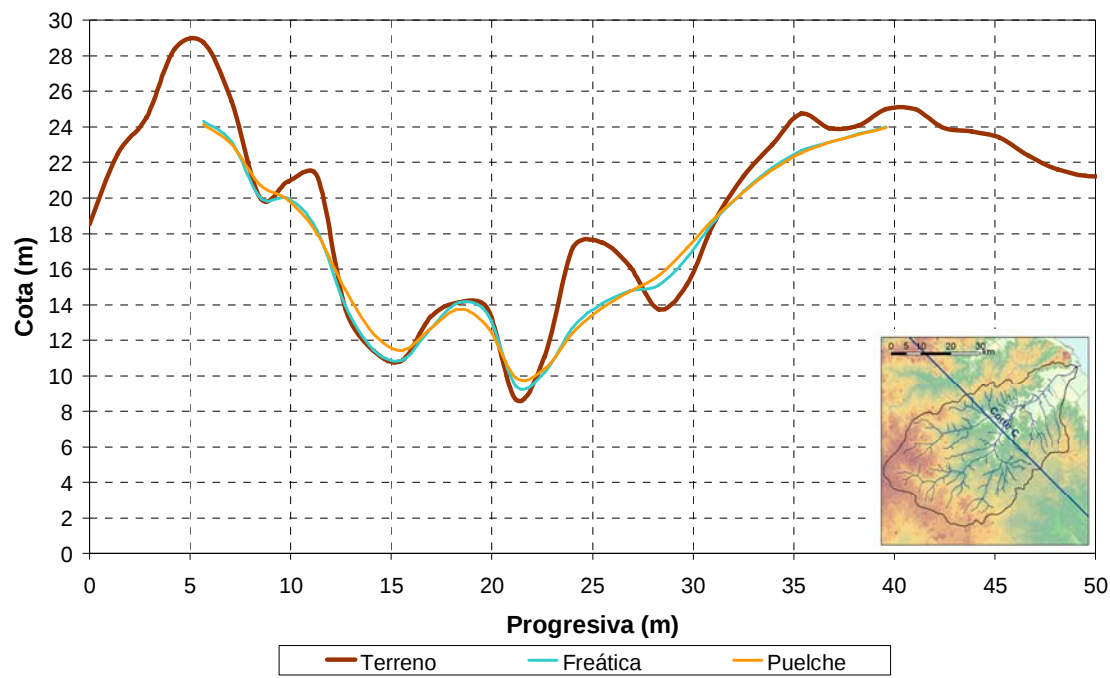
c) Corte C
