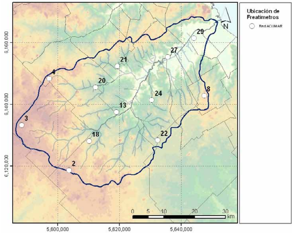
Figura 3.4.6. Ubicación de pozos de medición seleccionados
