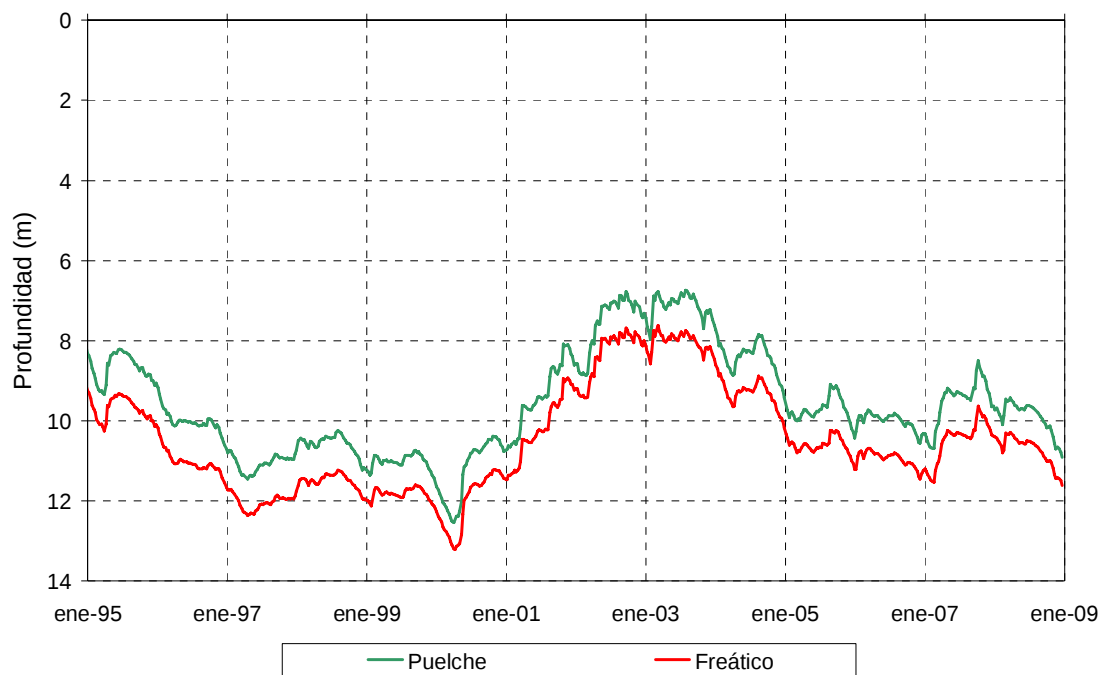
Figura 3.2.6. Sensibilidad de los niveles de agua subterránea a la conductividad horizontal del Puelche para el punto de control 'Pozo 13'.
