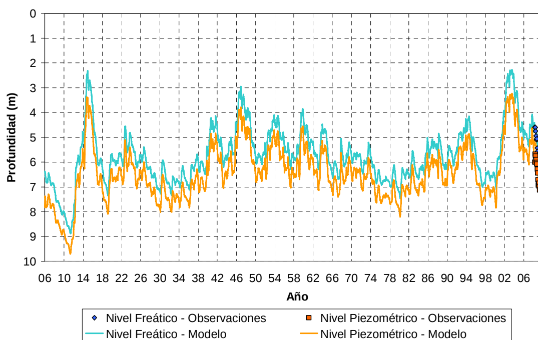
c) Niveles en Pozo 11
