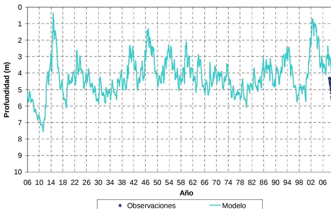
a) Nivel freático en Pozo 18
