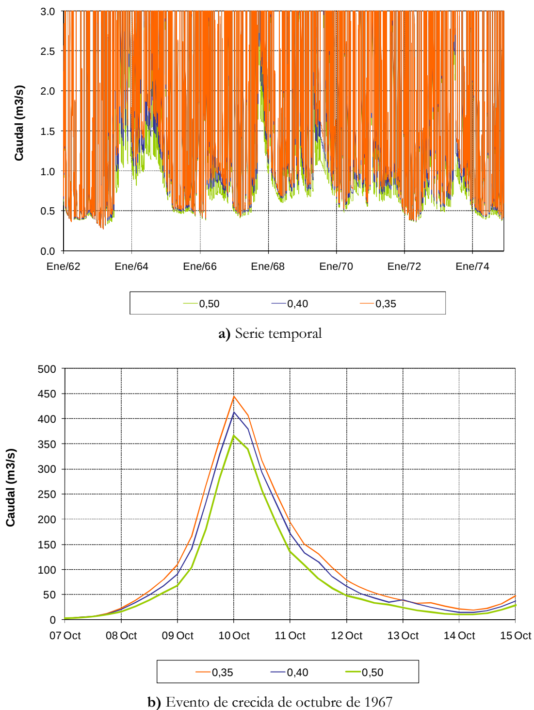
Figura 3.2.16. Caudal en Autopista Ricchieri para diferentes valores de la Humedad de Saturación.
