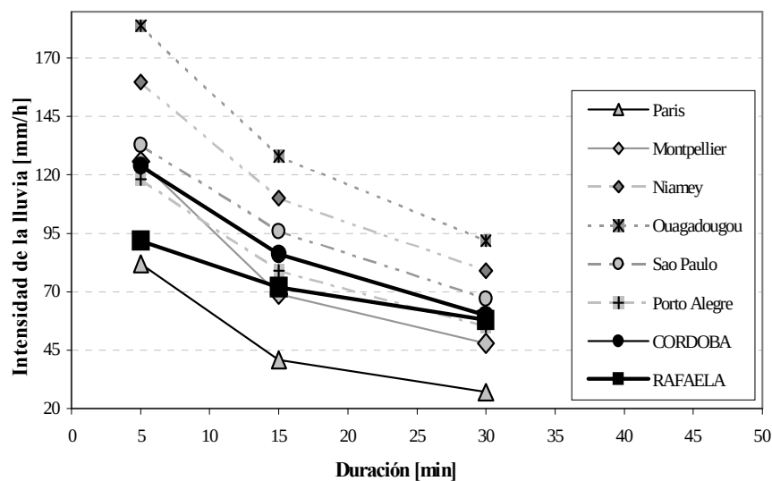
Figura 5.5. Curvas i-d-f correspondientes a ciudades de América Latina, África Occidental y Europa, para un tiempo de retorno, T_r = 2 años. (Fuentes: Bouvier, 1990; Tucci, 1993; Chocat, 1997b; Bertoni, 2001).
