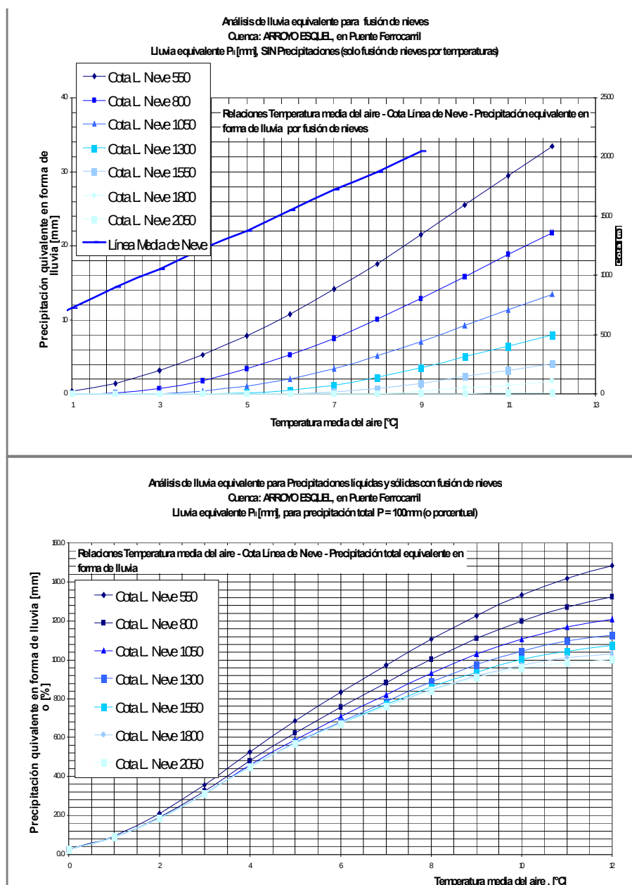
Figura 6.4. Lluvia equivalente, fusión de nieves y caudal máximo para la Cuenca del Arroyo Esquel, Chubut. (Fuente: Serra, 2002a).
