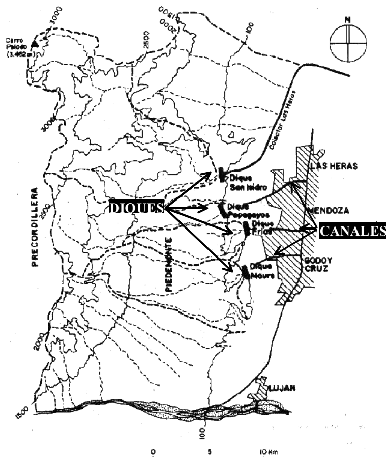
Figura 7.1. Pedemonte y conglomerado urbano del Gran Mendoza. Ubicación de diques aluvionales. (Fuente: INA-CRA).
