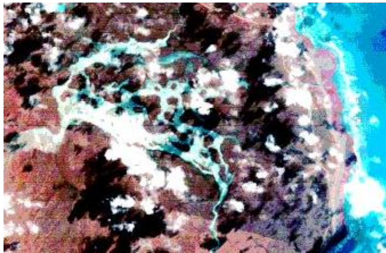
Figura 6.11. SIC Sistema Hidrológico Mixto Complejo: Cañadones y Urbanizaciones en Playa Magañas. Crecida extraordinaria del 24/25 de abril de 1998 y su descarga al mar. Las aguas que drenan de la alta meseta al Oeste, se concentran en la terraza intermedia en desordenados y erráticos encadenamientos lagunares para “cortar”, en su descarga al mar, las costas acantiladas compuestas de rodados patagónicos superficiales, estratos arenosos, areniscas y afloramientos de tobas más profundas.
