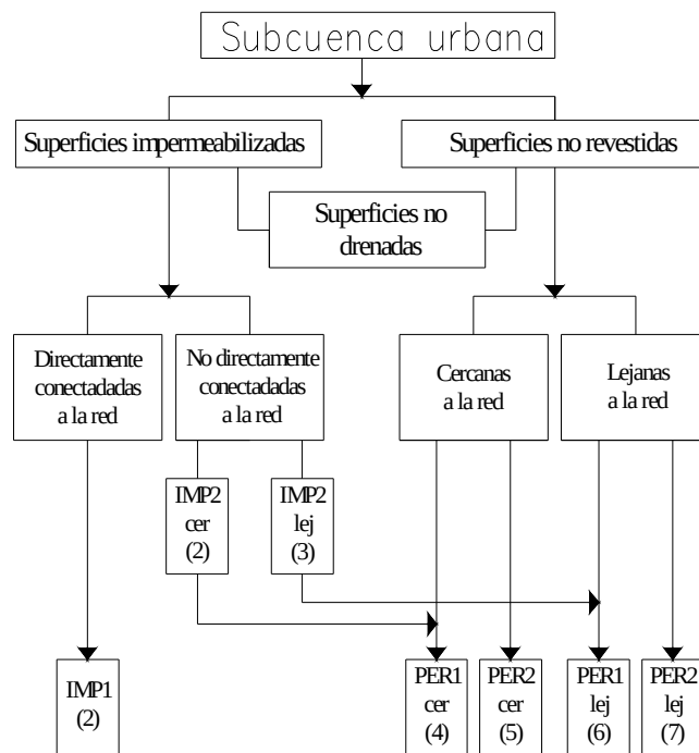
Figura 5.6. Clasificación de las superficies drenantes sobre una cuenca urbana (Bertoni, 2001).
