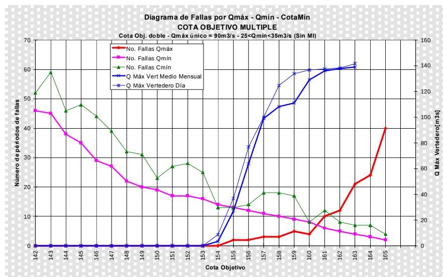
Figura 6.16. Embalse Ameghino: Diagrama de fallas para diferentes cotas objetivo.
