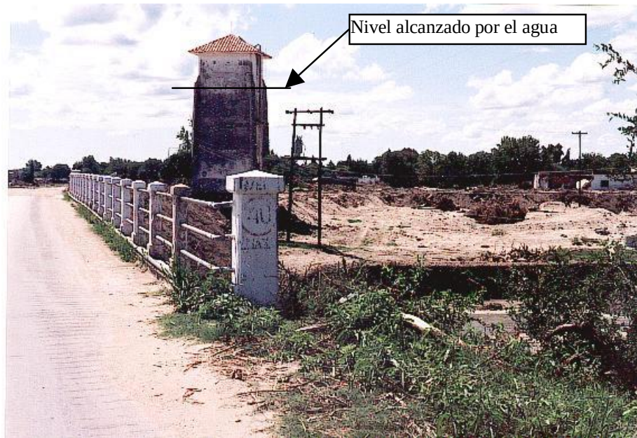
Foto 9.1. Sector inmediato aguas arriba del puente. Evento del 06/01/92 en S. C. Minas.
