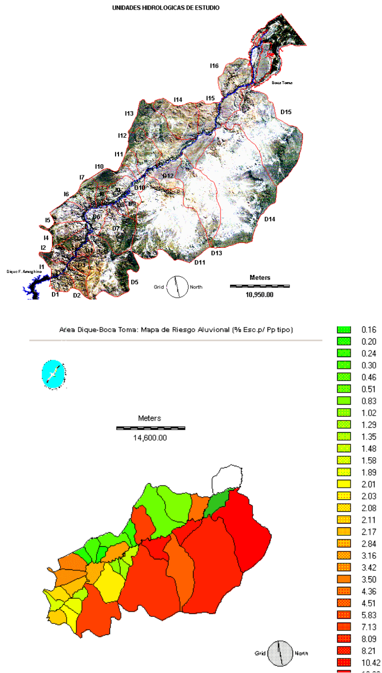
Figura 6.20. Mapa de Riesgo Aluvional (Área aluvional Dique-Boca Toma, VIRCh).
