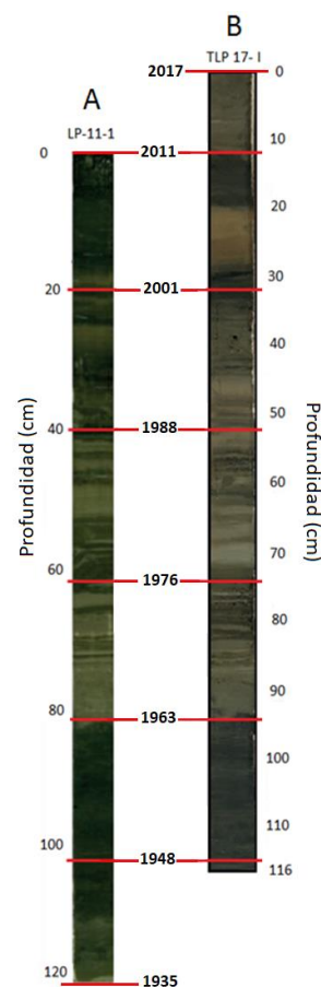
Figura 3. -Correlación de testigos LP-11-1 Stupar (2014) (A) y TLP-17-I (B) según tasas de sedimentación.
